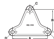
EQ-310
